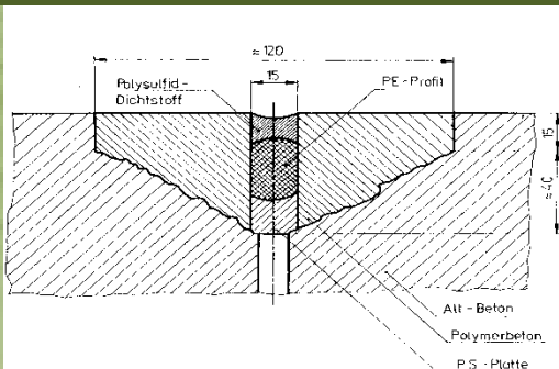
Betoninstandsetzung, Reprofilierung mit polymermodifizierten Mörtelsystemen
